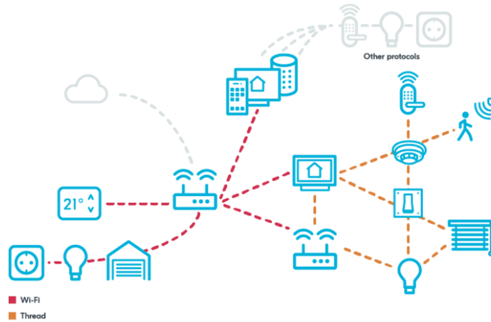
图 5 Matter 体系架构
